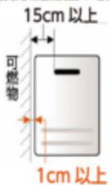
【側方近接設置の場合】
