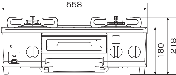
■外形寸法図 (単位:mm)
