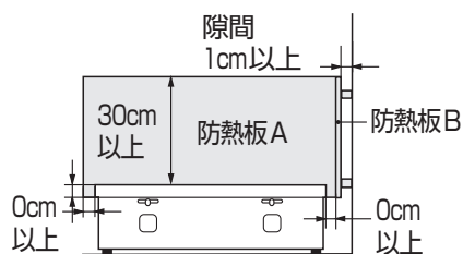
側面・背面
