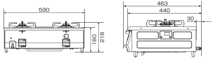
■外形寸法図(単位:mm)
