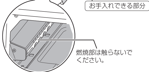
下火バーナー部拡大図
