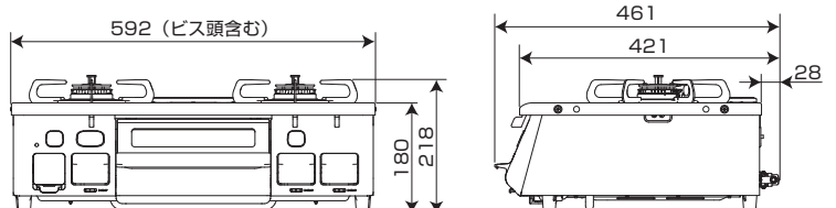
■外形寸法図 (単位: mm)
