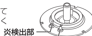
電極（点火プラグ）
