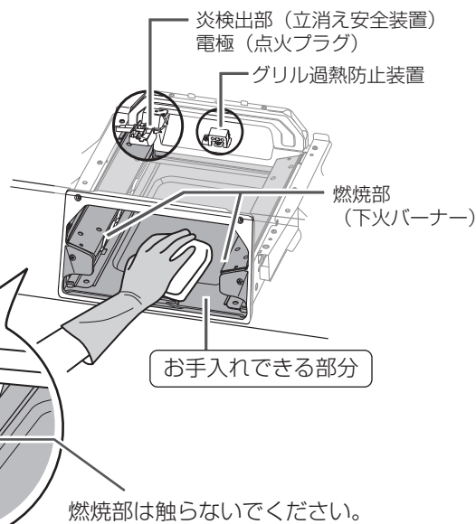
下火バーナー部拡大図
