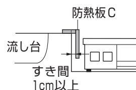
流し台などの側面
