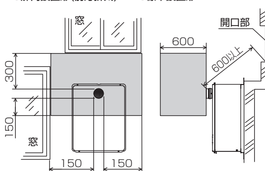
PS扉内設置形(前方排気)・PS標準設置形
