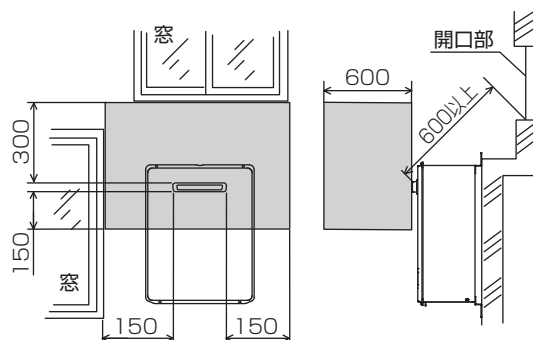
屋外壁掛設置形
