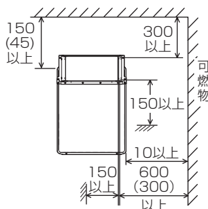
屋外壁掛設置形に側方排気カバーを取り付ける場合
