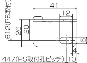
PS取付板下 (左右対称形状。本図は右を示す)
