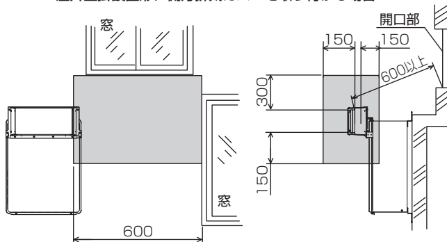
屋外壁掛設置形に側方排気カバーを取り付ける場合
