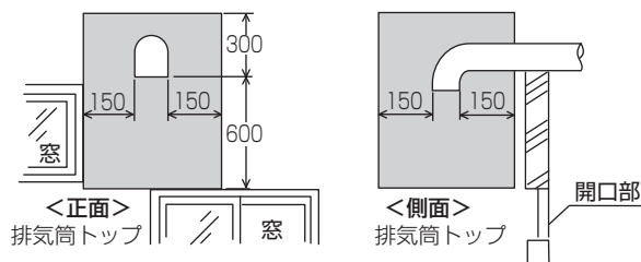
PS扉内設置形(後方/上方排気延長)を排気延長した場合の排気トップ部
