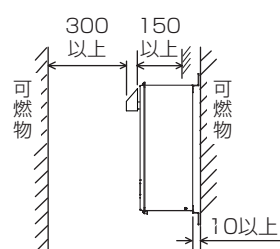
屋外壁掛設置形に上方排気カバーを取り付ける場合
