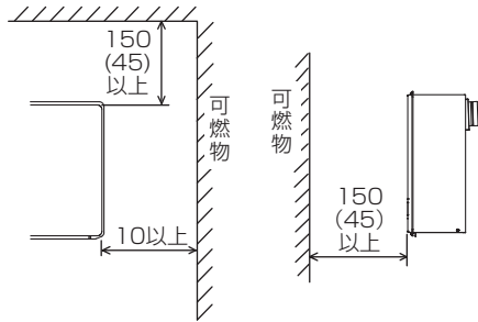
PS扉内設置形(後方排気延長)
