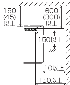
屋外壁掛設置形に上方排気カバーを取り付ける場合
