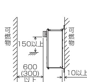
PS扉内設置形(前方排気)・PS標準設置形
