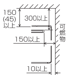
屋外壁掛設置形
