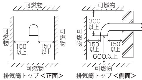
PS扉内設置形(後方/上方排気延長)を 排気延長した場合の排気口出口
