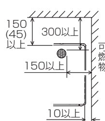
PS扉内設置形(前方排気)・PS標準設置形
