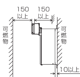
屋外壁掛設置形に側方排気カバーを取り付ける場合
