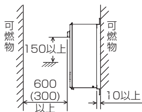
屋外壁掛設置形に側方排気カバーを取り付ける場合
