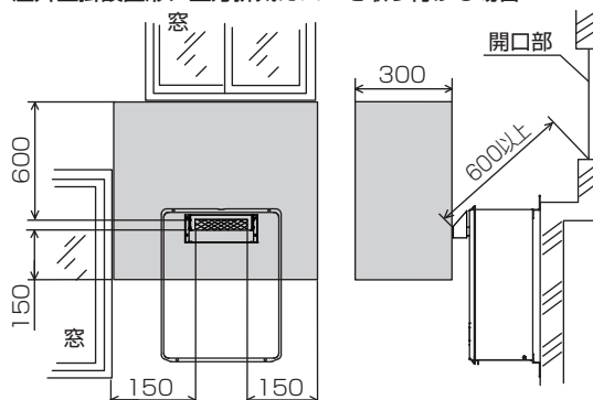
屋外壁掛設置形に上方排気カバーを取り付ける場合
