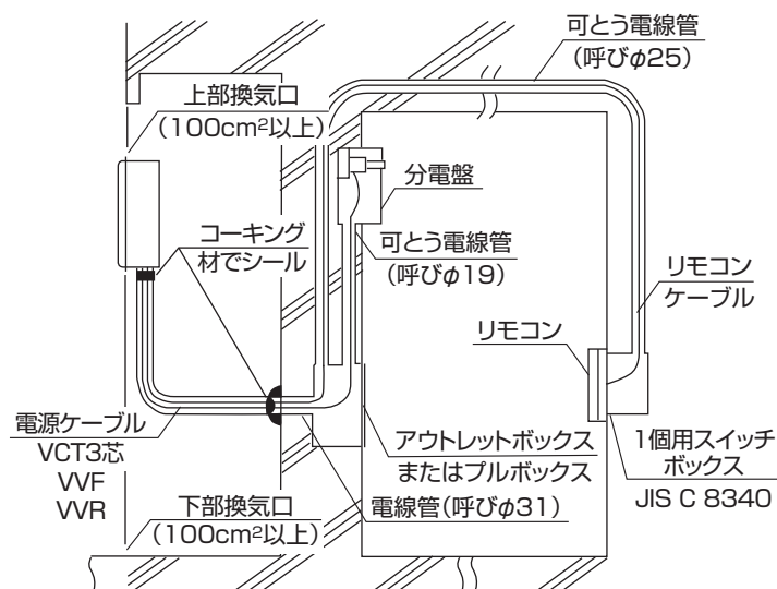
アース線付き電源ケーブルの接続位置
