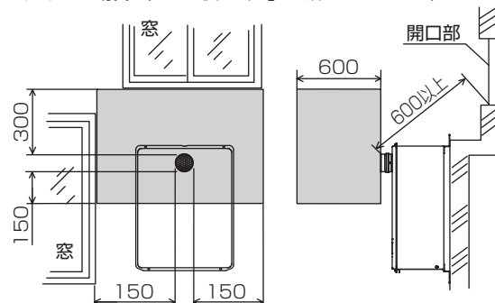
Tタイプの場合（FHの後ろが「E」で始まるシリーズ）
