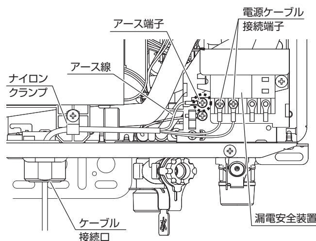
アース線付き電源ケーブルの接続位置
