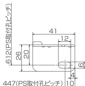
PS取付板下(左右対称形状。本図は右を示す)
