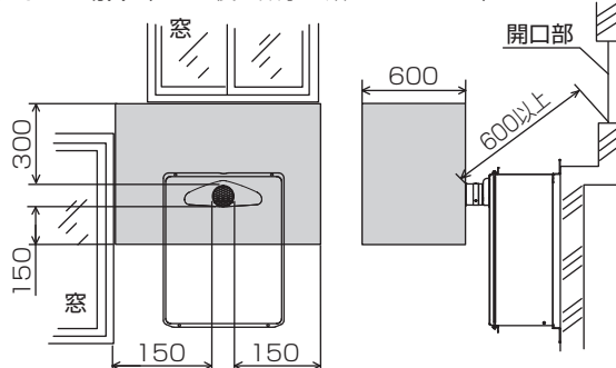
Tタイプの場合（FHの後ろが数字で始まるシリーズ）
