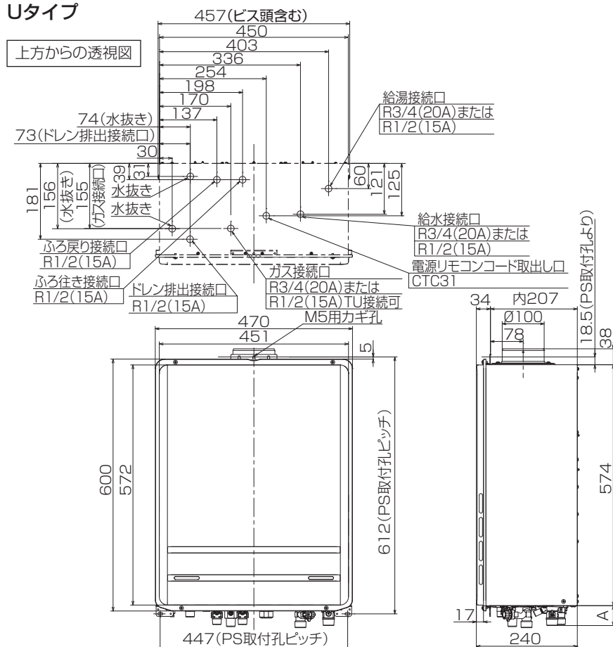
機器底面より各接続口までの寸法
