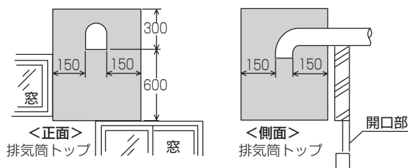
T2・B・Uタイプを排気延長した場合の排気口出口
