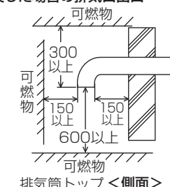
T2・B・Uタイプを排気延長した場合の排気口出口
