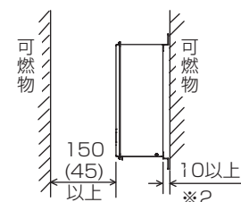
B・Uタイプの場合 [※1：Bタイプのみ、※2：Uタイプのみ]
