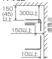
Wタイプの場合
