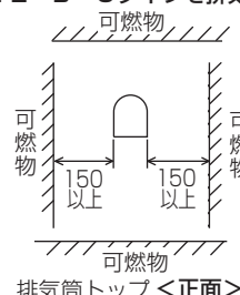
T2・B・Uタイプを排気延長した場合の排気口出口
