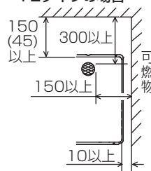
T・T2タイプの場合
