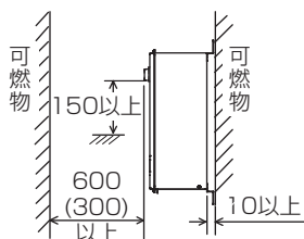
B・Uタイプの場合 [※1：Bタイプのみ、※2：Uタイプのみ]
