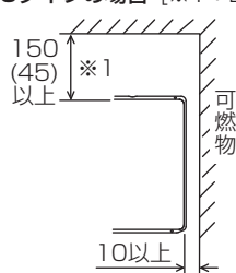
B・Uタイプの場合 [※1：Bタイプのみ、※2：Uタイプのみ]
