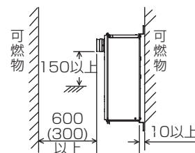
T2・B・Uタイプを排気延長した場合の排気口出口
