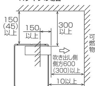
Aタイプの場合
