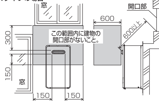
T2・B・Uタイプを排気延長した場合の排気口出口
