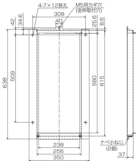
TBFH-S1(パイプシャフト開口幅342mm用)
