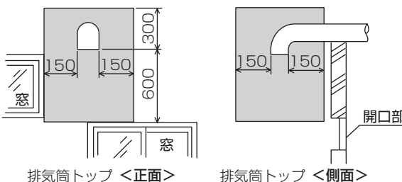
T2・B・Uタイプを排気延長した場合の排気口出口
