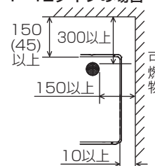
T2・B・Uタイプを排気延長した場合の排気口出口
