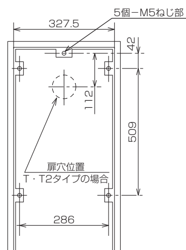
TBFH-SW用 (W-662)
