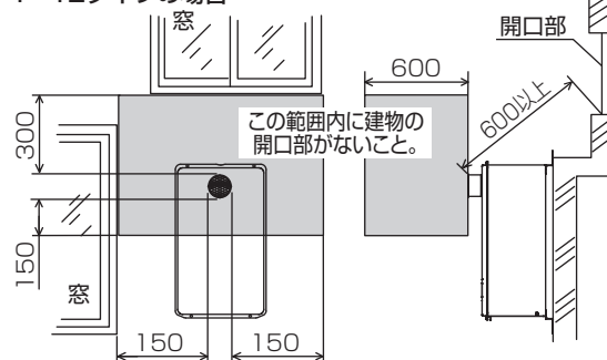
T・T2タイプの場合
