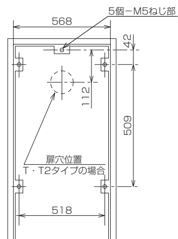
TBFH-S2用 (W-550)
