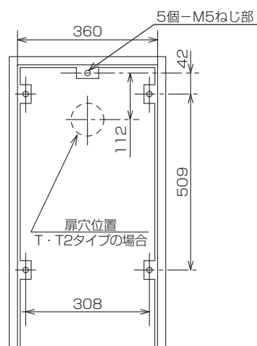
TBFH-S1用 (W-342)
