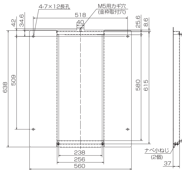
TBFH-S2(パイプシャフト開口幅550mm用)
