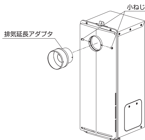
T2タイプの場合
