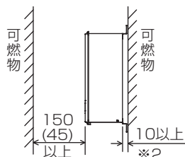
B・Uタイプの場合 ※1：Bタイプのみ、※2：Uタイプのみ
