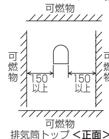
T2・B・Uタイプを排気延長した場合の排気口出口
