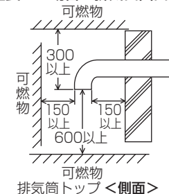
T2・B・Uタイプを排気延長した場合の排気口出口
