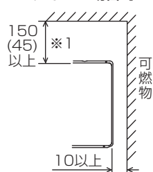
B・Uタイプの場合 ※1：Bタイプのみ、※2：Uタイプのみ
