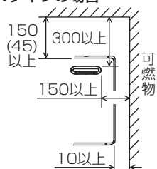
B・Uタイプの場合 ※1：Bタイプのみ、※2：Uタイプのみ
