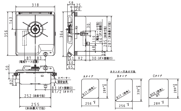
※本体のスペーサー位置を変更することによりA、B、Cタイプに対応できます。
