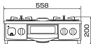
外形寸法 (単位: mm)
