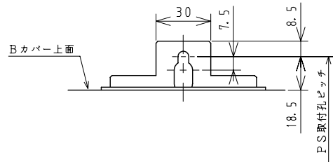
M5 カギ孔部詳細図
