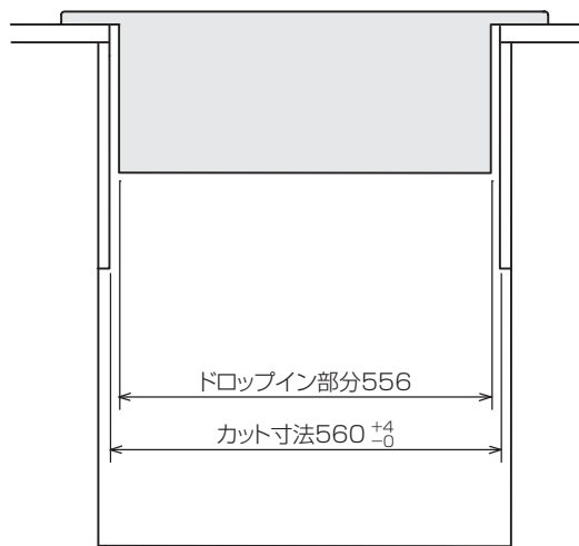
正面図
