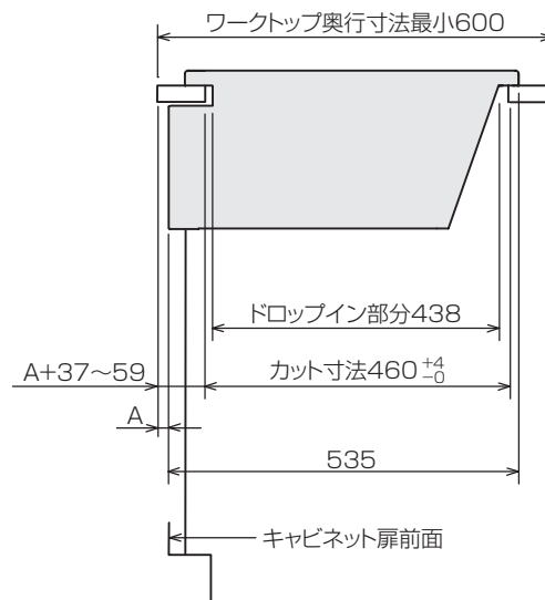
側面図
