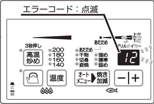
※図は強火力バーナーが右側の機器の場合です。
