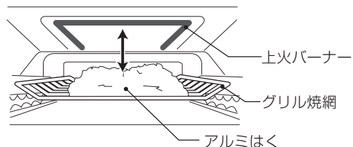
<グリル庫内を正面から見た図>
