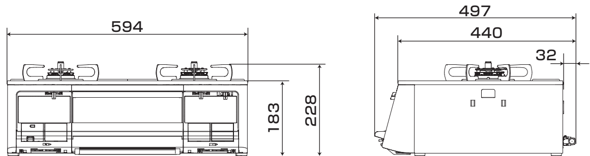
外形寸法図（単位：mm）
