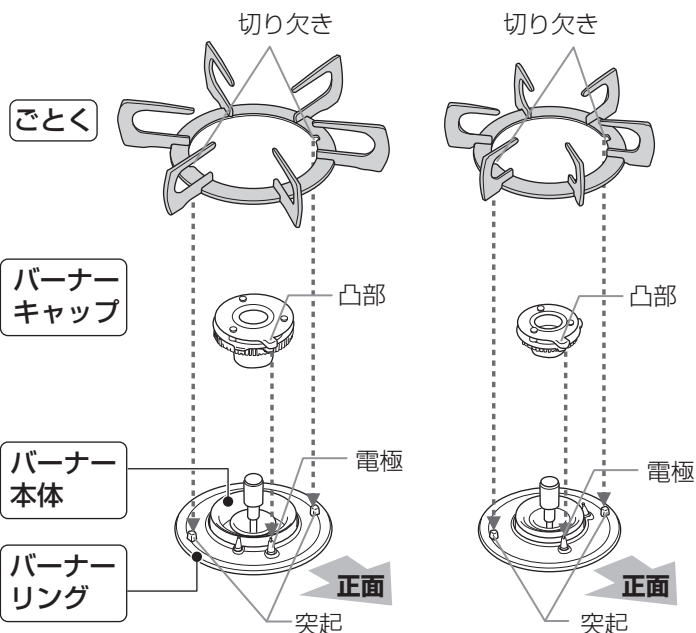
標準バーナー・強火力バーナー
